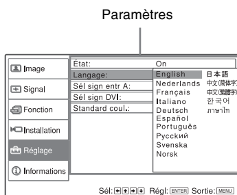
Menu local
