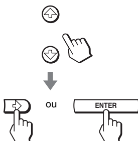
Menu local
